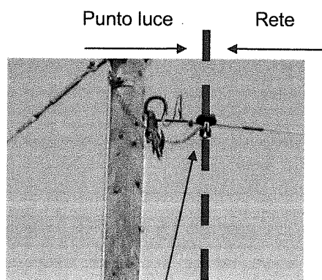
Morsetti (esterni)
