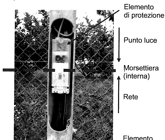
Punto luce
